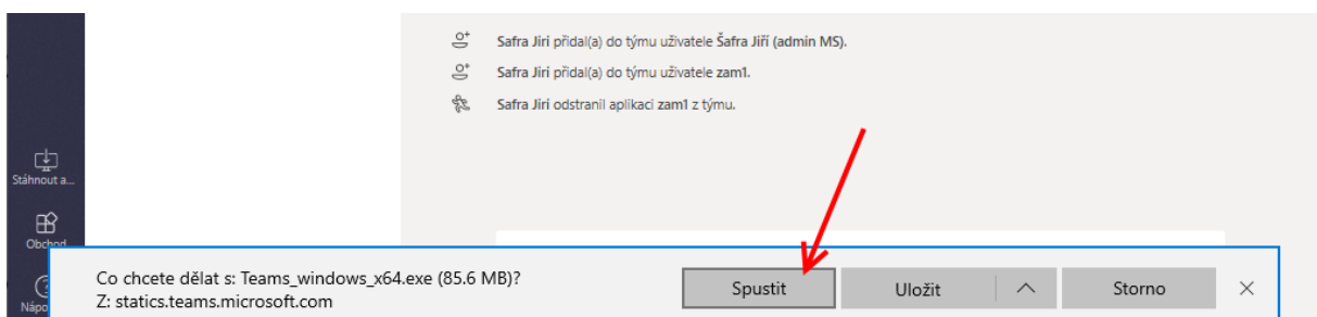
Obr. 11 Spuštění instalátoru
