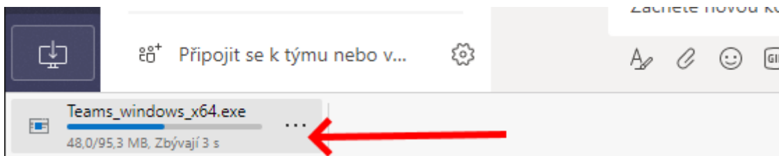
Obr. 10 Stahovaný instalátor
